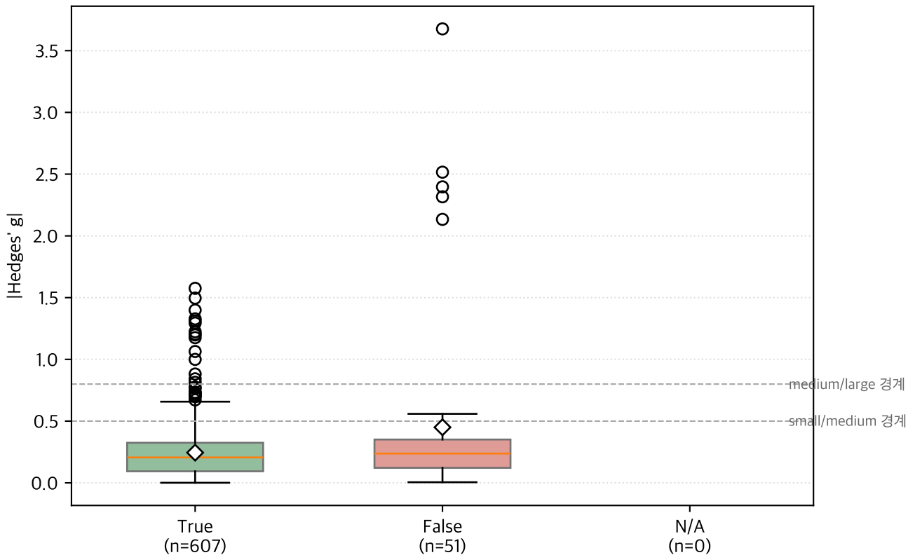
plan-level effect size 분층 — anchor=B1 의 |g| 분포 by plan 회복 여부 (3 평면 통합)
