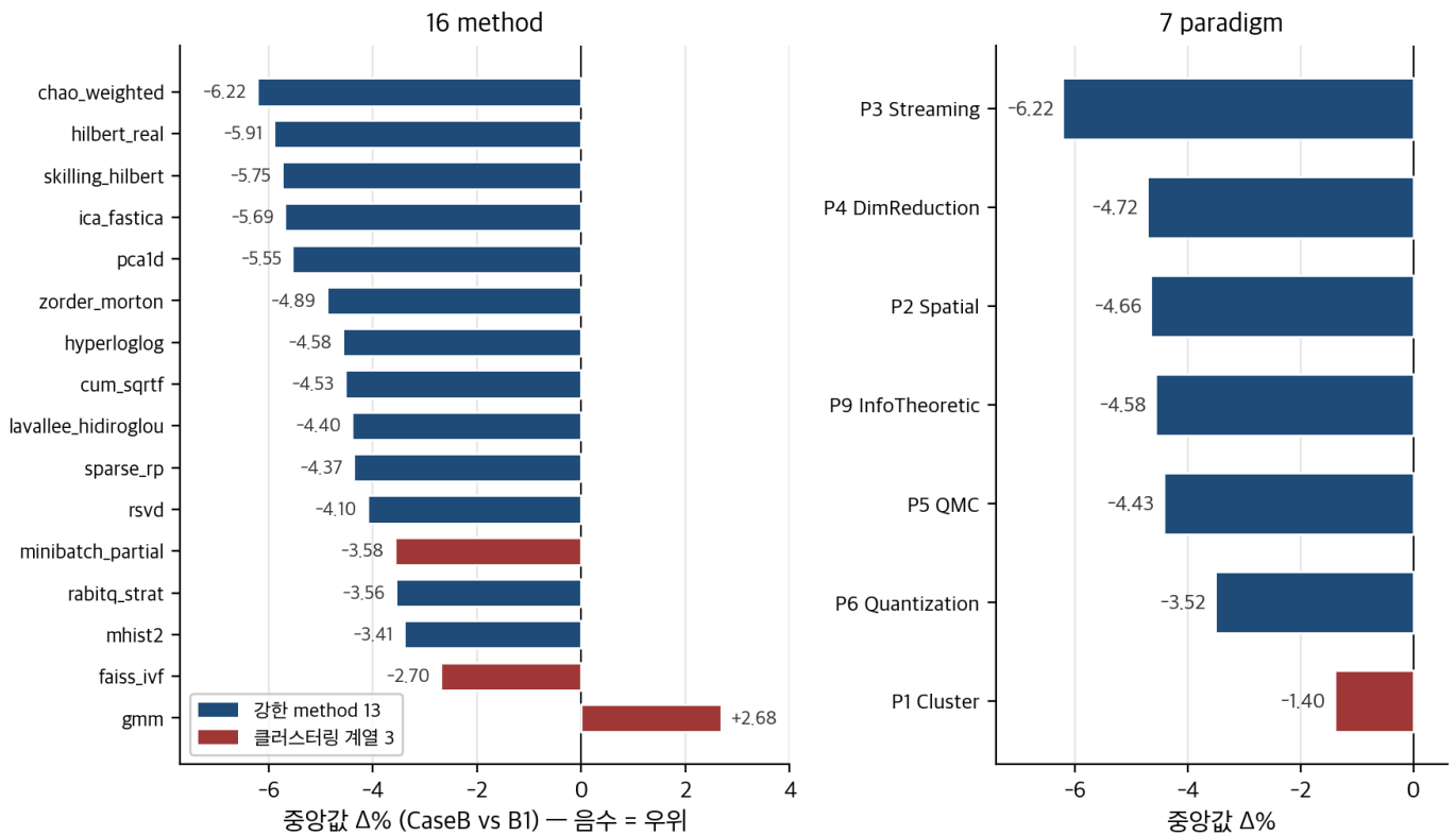
그림 4-1. method·paradigm별 CaseB vs B1 중앙값 Δ% — 16 method와 7 paradigm. 강한 13개와 클러스터링 3개를 색으로 구분.
