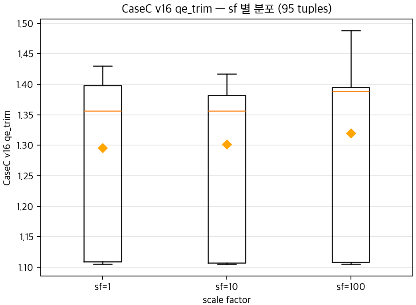
그림 4-2A·B. v16 95 tuple 전수 측정. (A) paired \Delta\% vs B1 — 95/95 = 100% 음수, 중앙값 -11.32%. (B) sf 별 qe_trim 분포 — sf=1·10·100 의 mean 차이 작음 (1.296/1.301/1.320).
