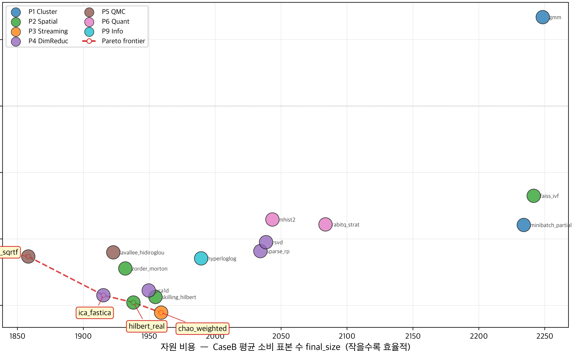
자원·정확도 Pareto frontier — 자원 = 소비 표본 수 (final_size)
