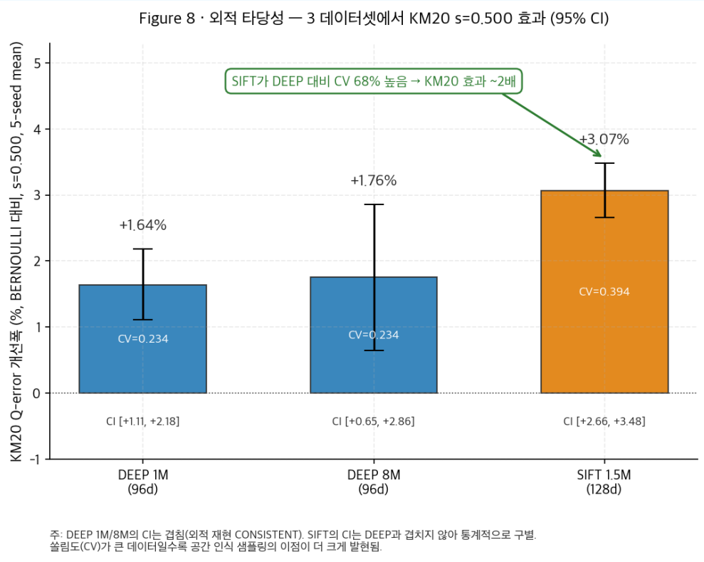
외적 타당성 — DEEP 1M / 8M / SIFT 1.5M, KM20 s=0.500 효과 95% CI
