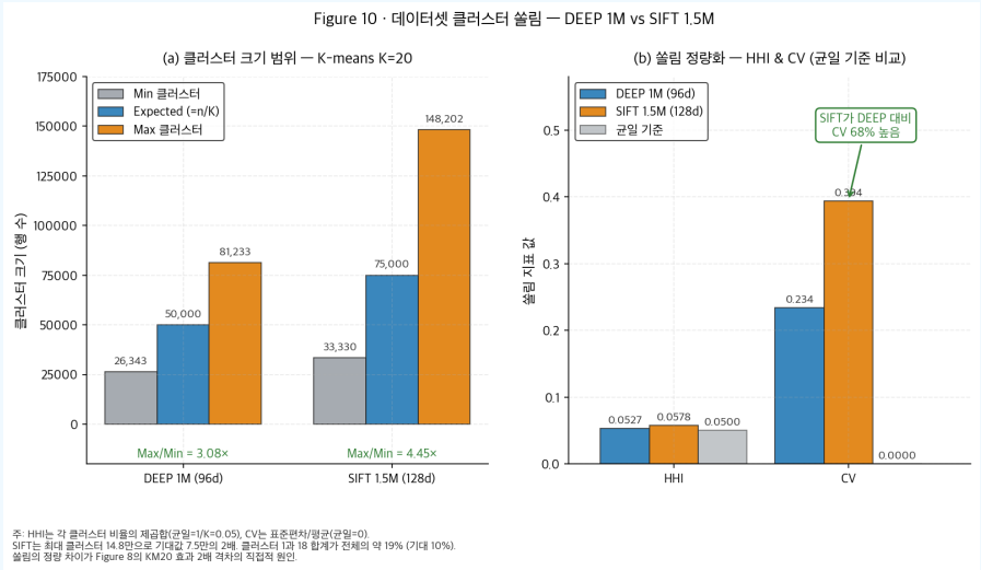
클러스터 쓸림도 — DEEP CV 0.234 vs SIFT CV 0.394 (HHI 정량)
