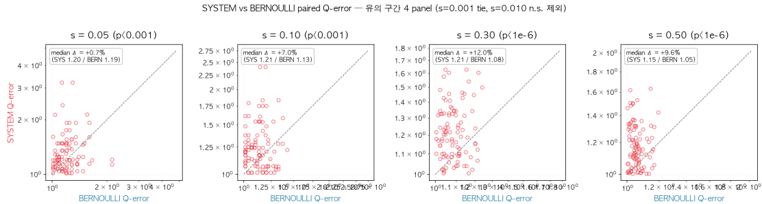
그림 3. SYSTEM ↔ BERNOULLI paired Q-error 의 4 selectivity panel (s = 0.05 / 0.10 / 0.30 / 0.50)
