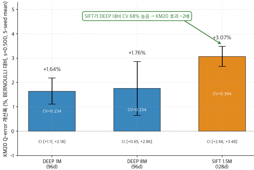
Figure 8 · 외적 타당성 — 3 데이터셋에서 KM20 s=0.500 효과 (95% CI)
