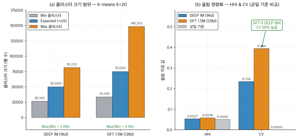
Figure 10 · 데이터셋 클러스터 쏠림 — DEEP 1M vs SIFT 1.5M
