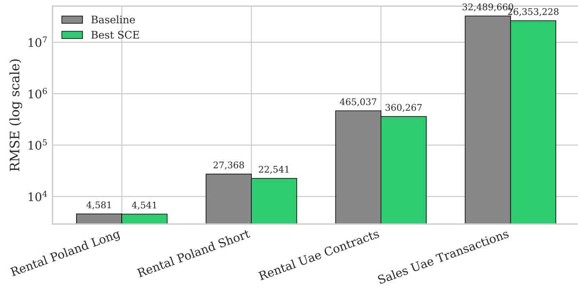
RMSE: Baseline vs Best SCE
