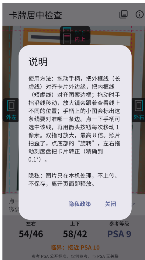
图 11 说明对话框
