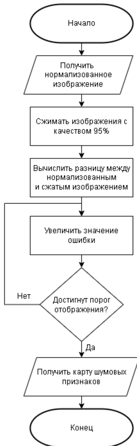
Рисунок 2.3 – Алгоритм извлечения признаков.
