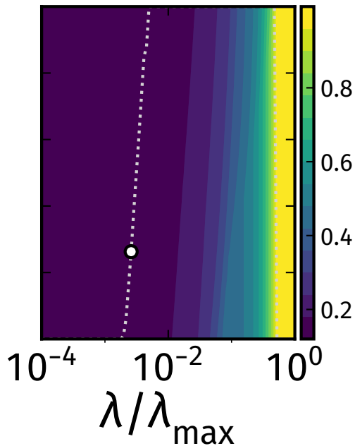
eunite2001
