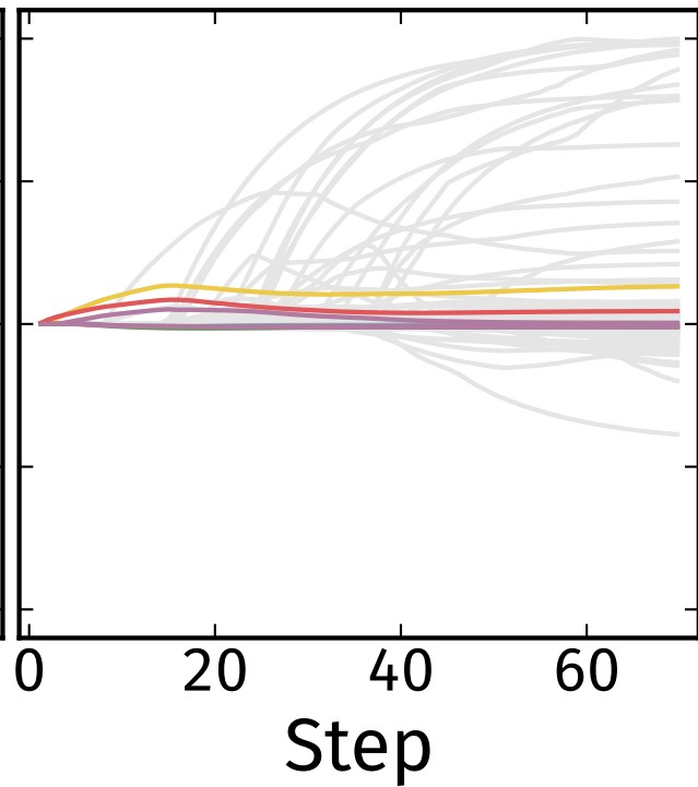
Max-Abs
