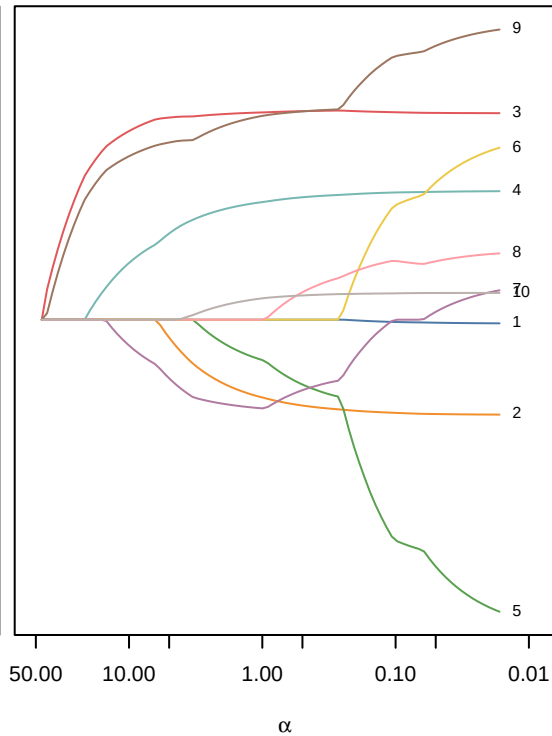
Lasso
