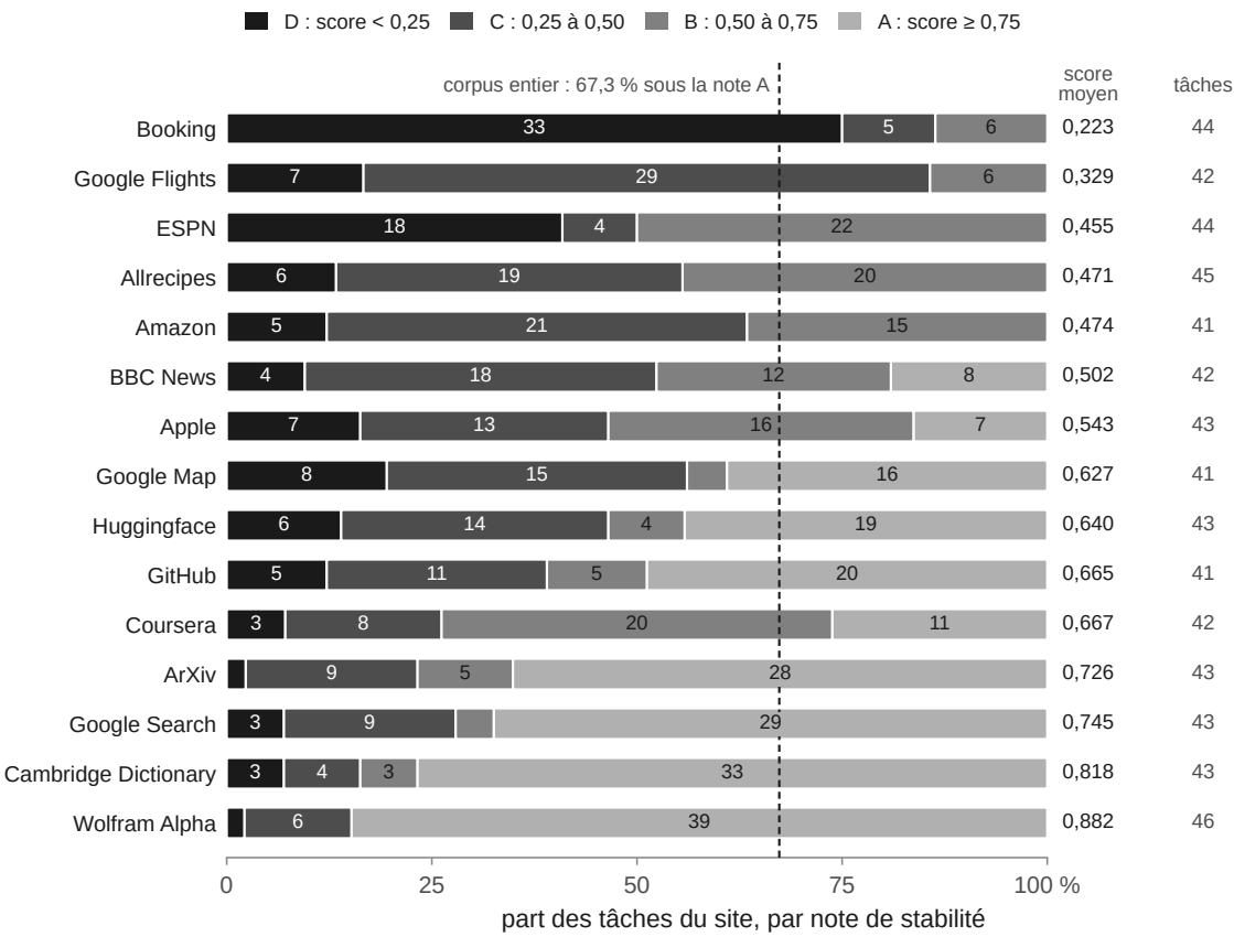
Figure 1. Décadence par site : les 643 tâches de WebVoyager notées au 15 août 2026
