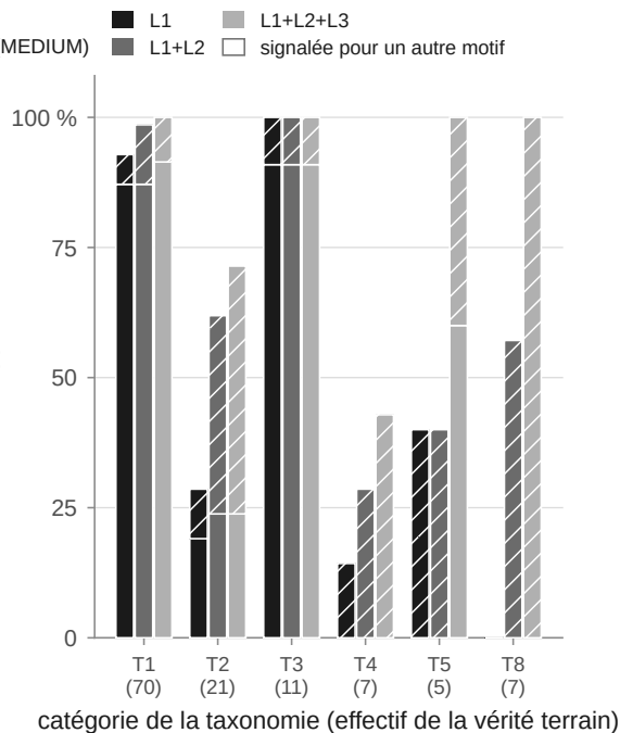
(b) rappel par catégorie, seuil intermédiaire (MEDIUM)
