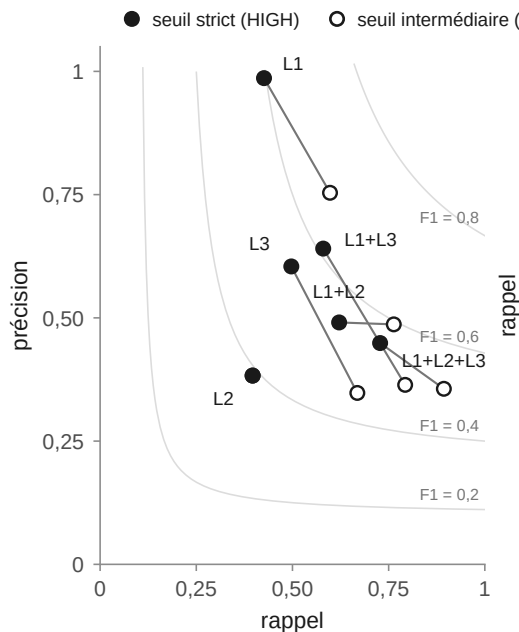
(a) plan précision-rappel
