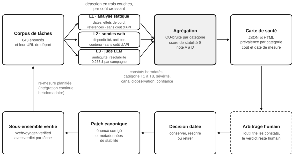
Figure 7. Architecture fonctionnelle de benchmark-doctor
