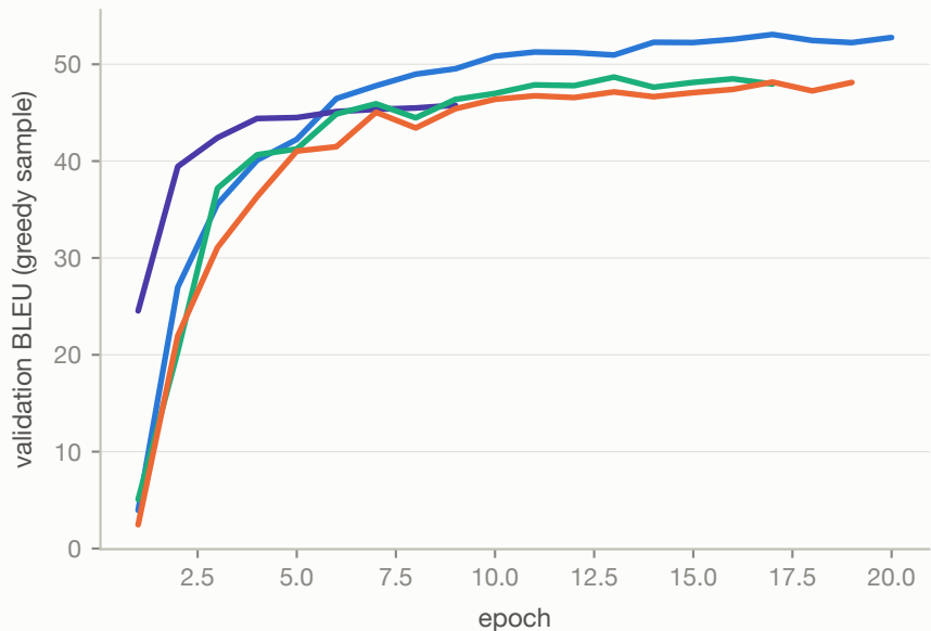
Validation BLEU
