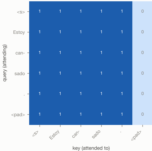
Padding mask
