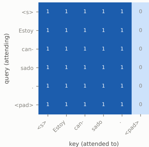
Padding mask
