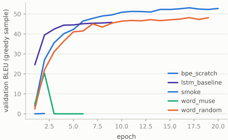
Validation BLEU
