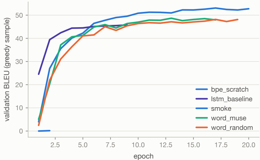
Validation BLEU
