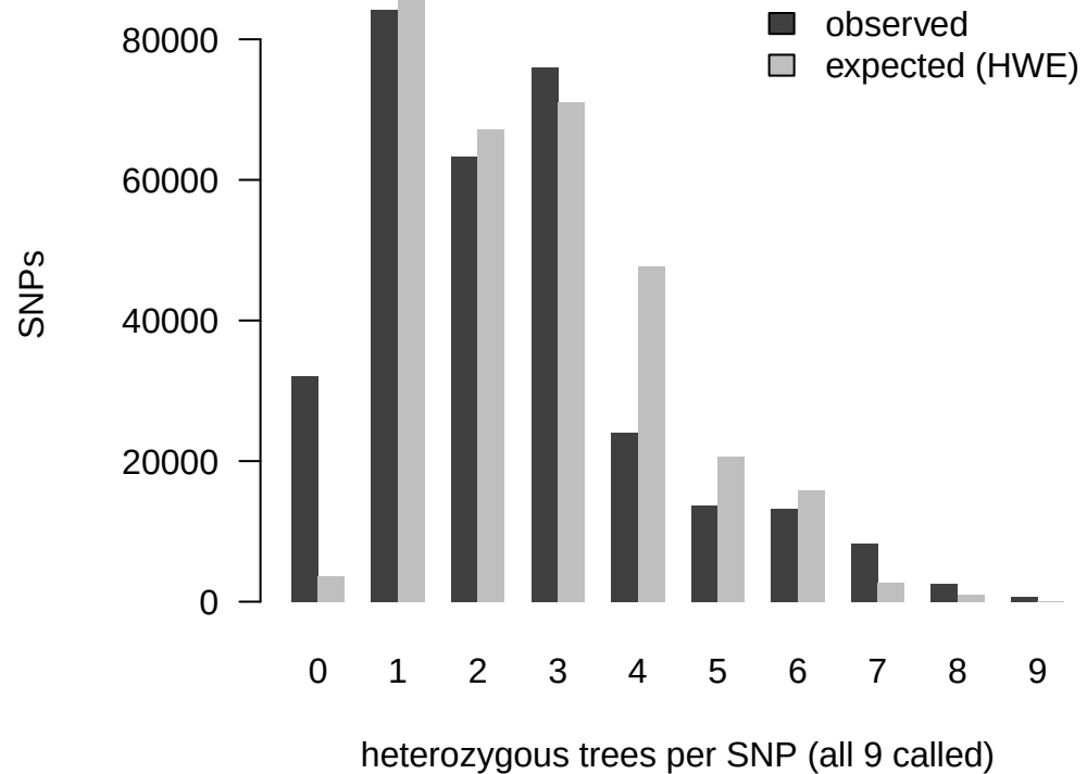
d20_v2_G1: observed vs HWE
