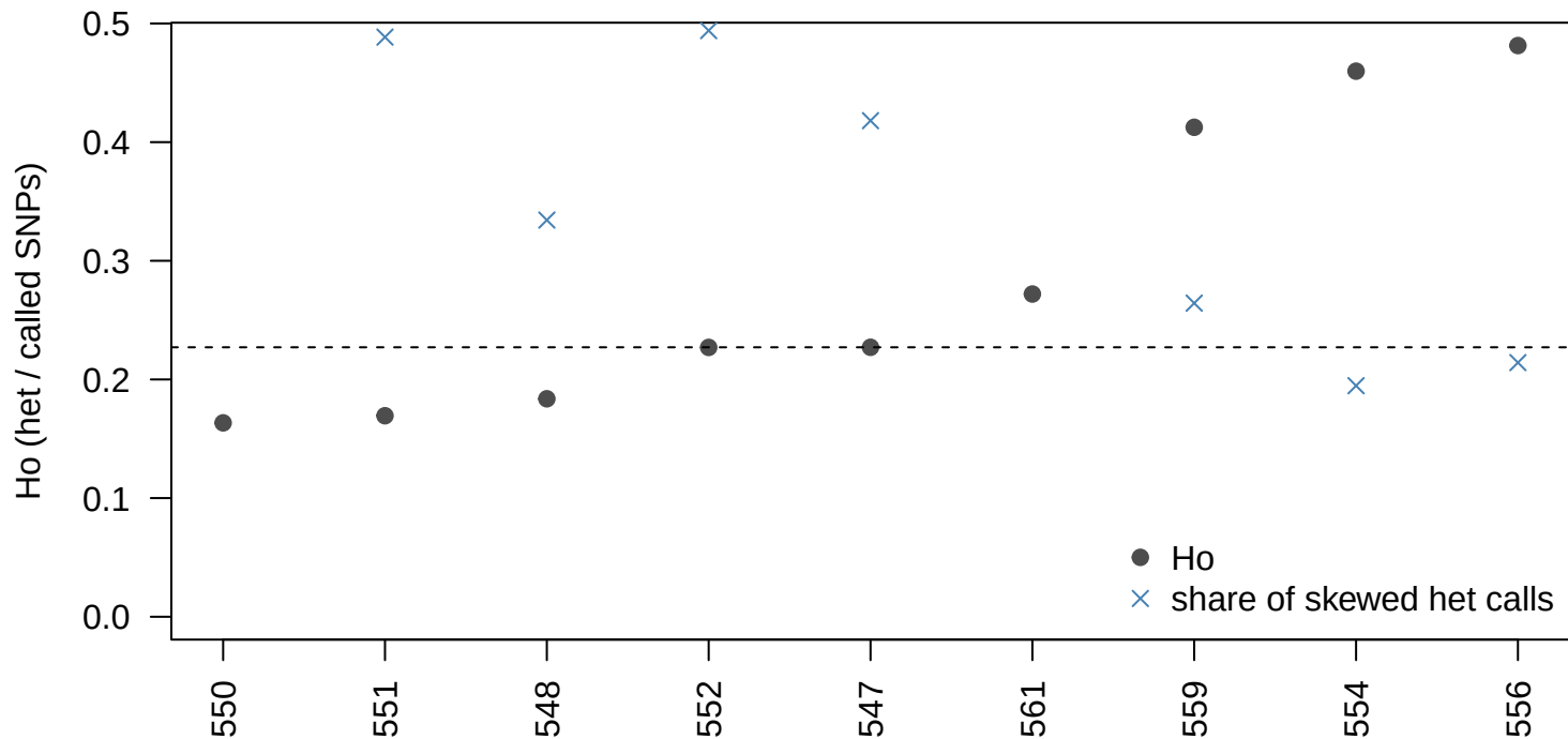
d20_mask_win1kb: Ho per tree (red = >3 MAD)
