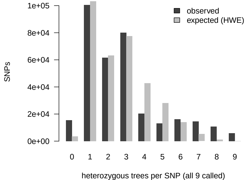
d20_mask_ab: observed vs HWE
