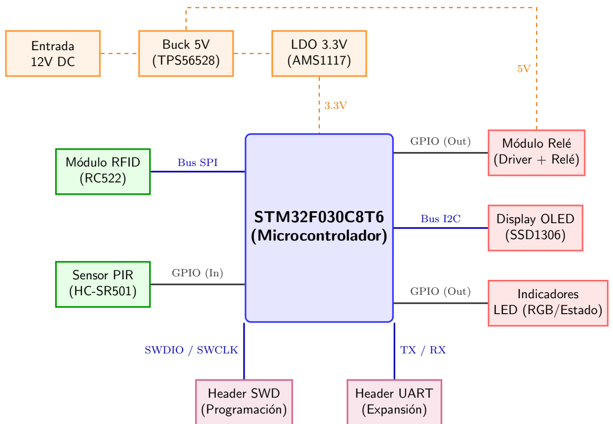
Figura 1: Diagrama de bloques general de la arquitectura de hardware del sistema. Se ilustra el flujo de señales de datos (SPI, I2C, UART), señales de control (GPIO) y las principales vías de distribución de energía.
