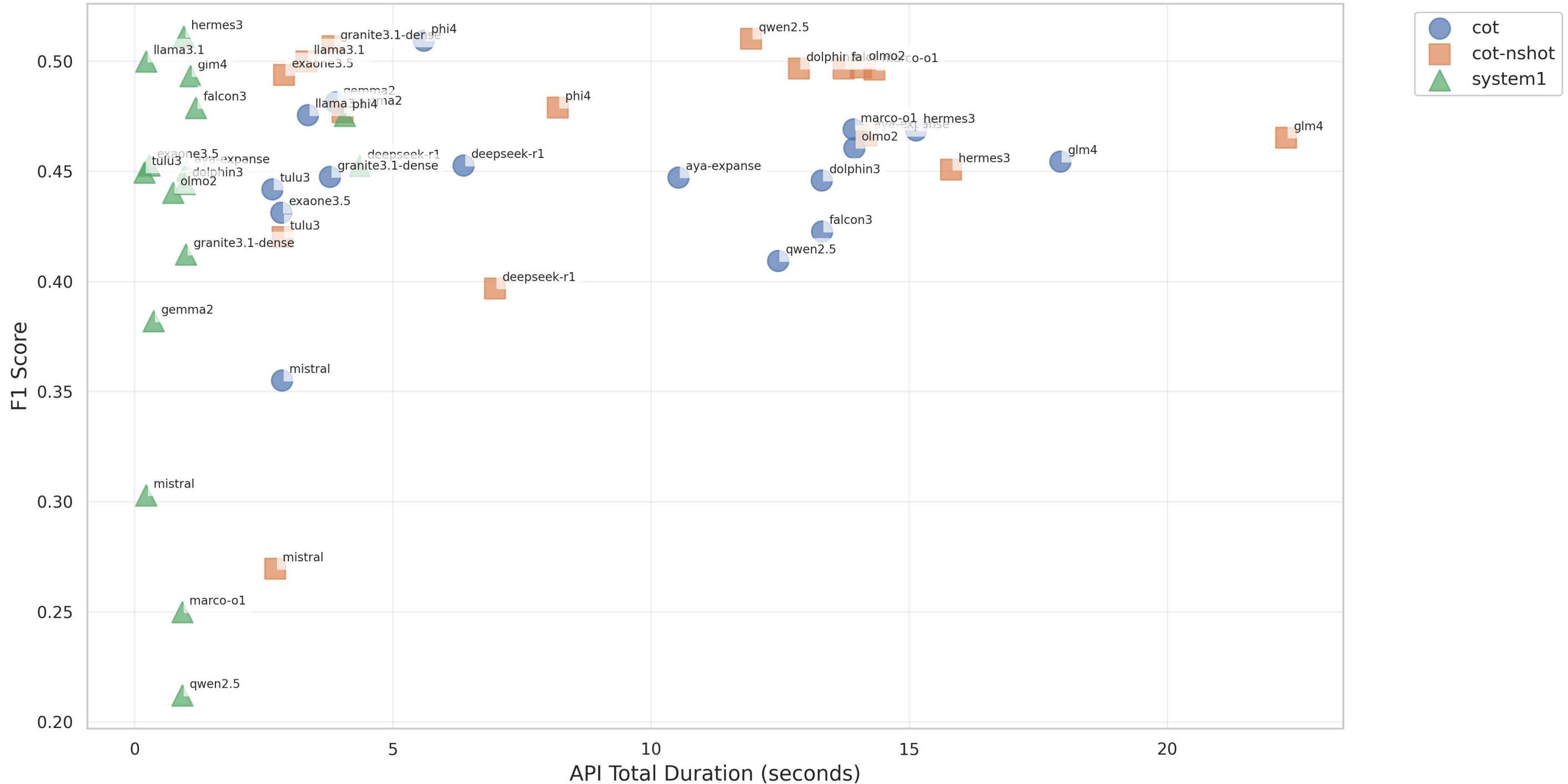
F1 Score vs API Total Duration (seconds) (StandardLLM)
