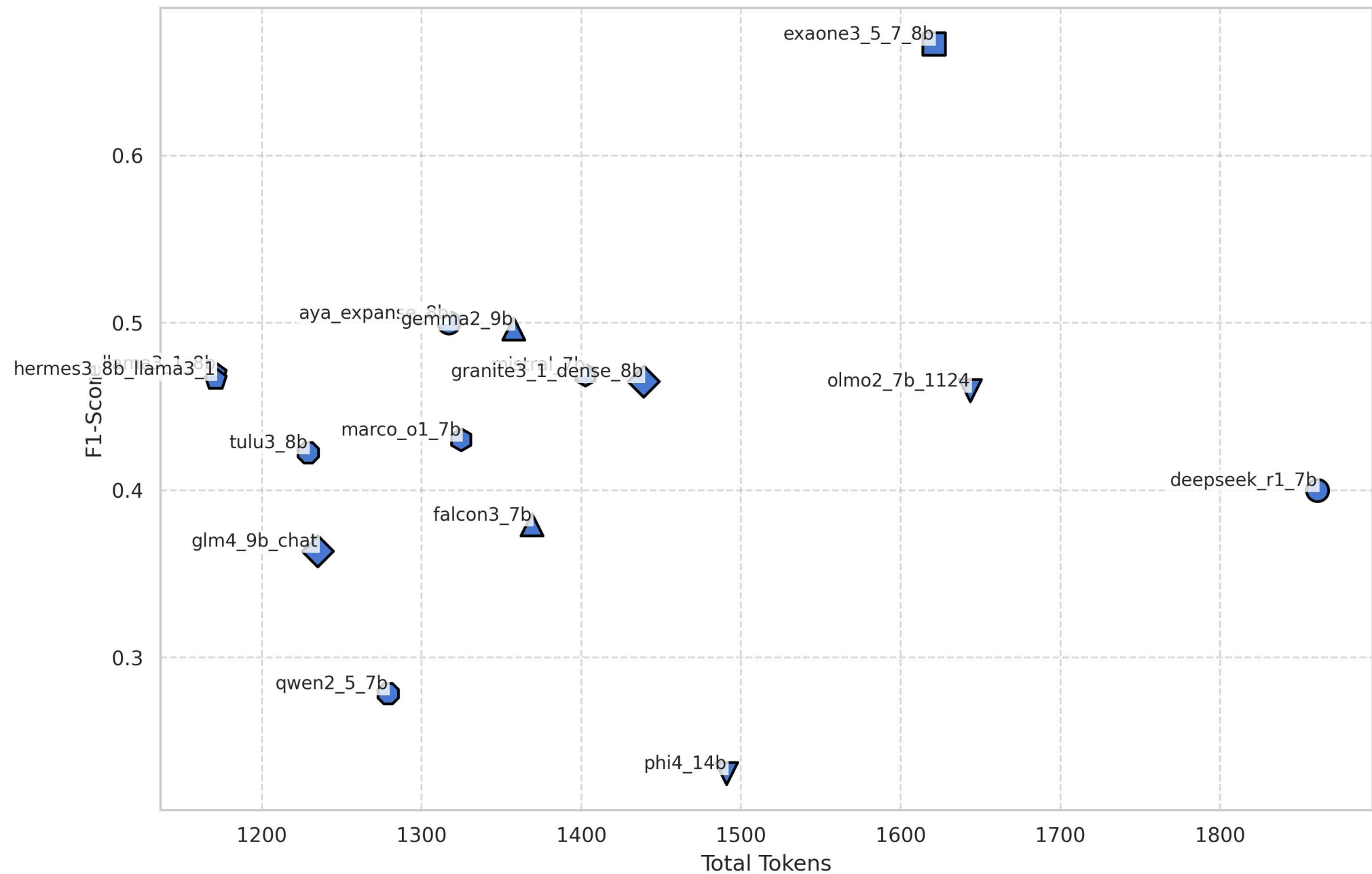
F1-Score vs Total Tokens (AgenticSimLLM)
