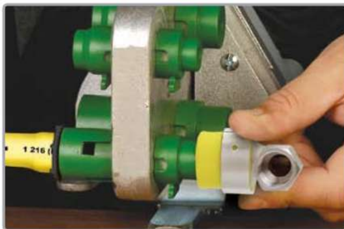
Segunda termofusión
