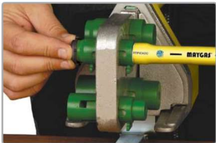
Primera termofusión
