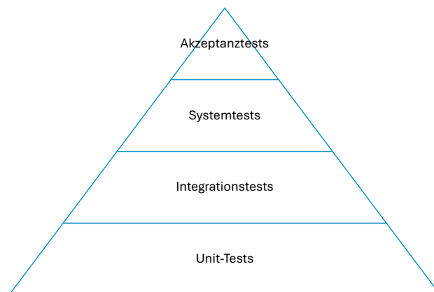
Abbildung 2.1: Testpyramide nach [10]
