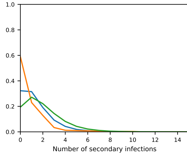
Poisson
