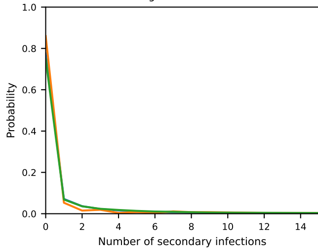
Negative Binomial
