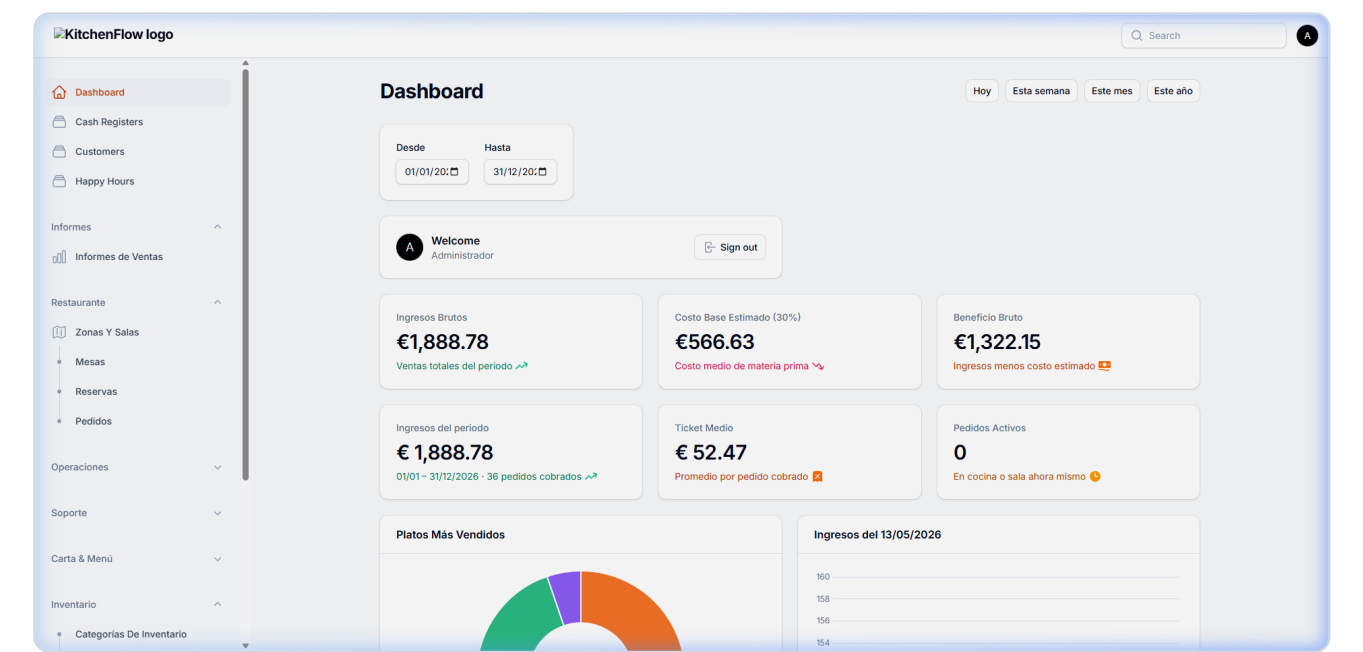
Figura 4: Dashboard Principal del ERP con analíticas diarias, ocupación física y ventas.
