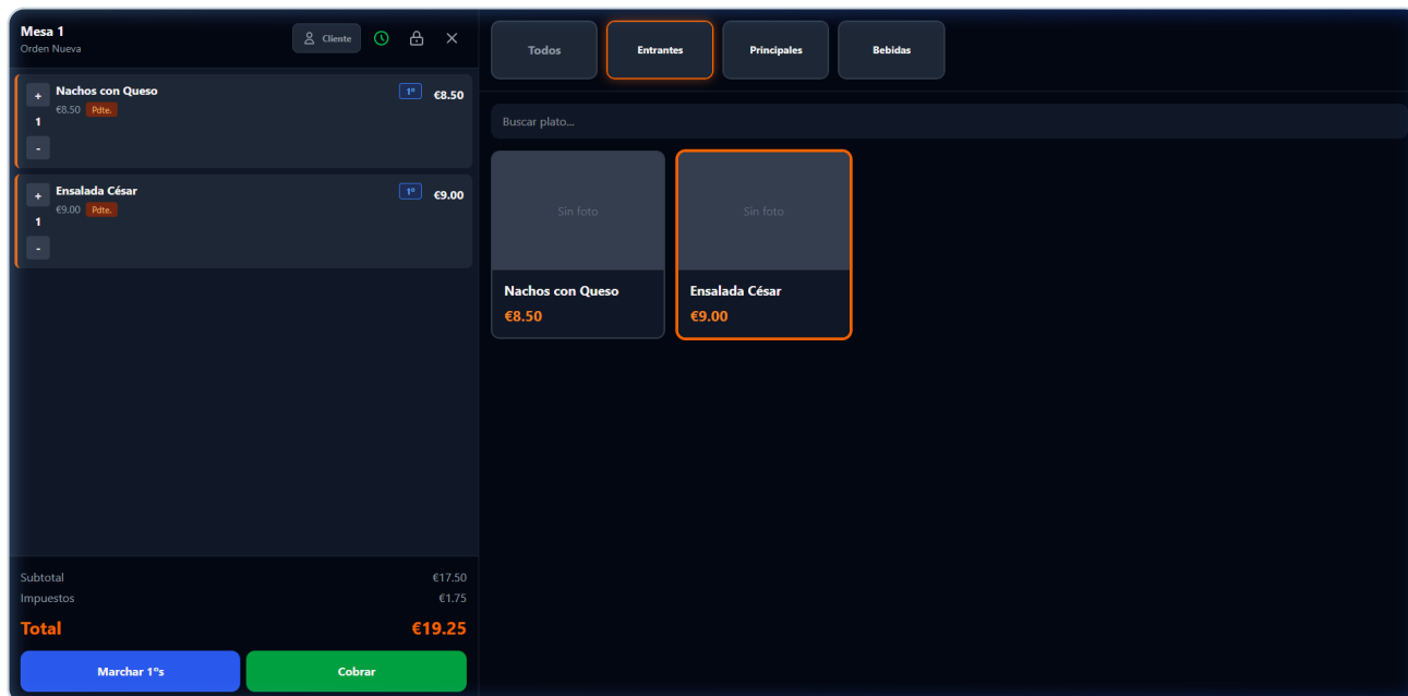
Figura 2: Carrito interactivo del POS con selección de cursos (Primeros/Segundos) y envío síncrono.
