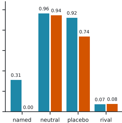
Qwen3-4B
