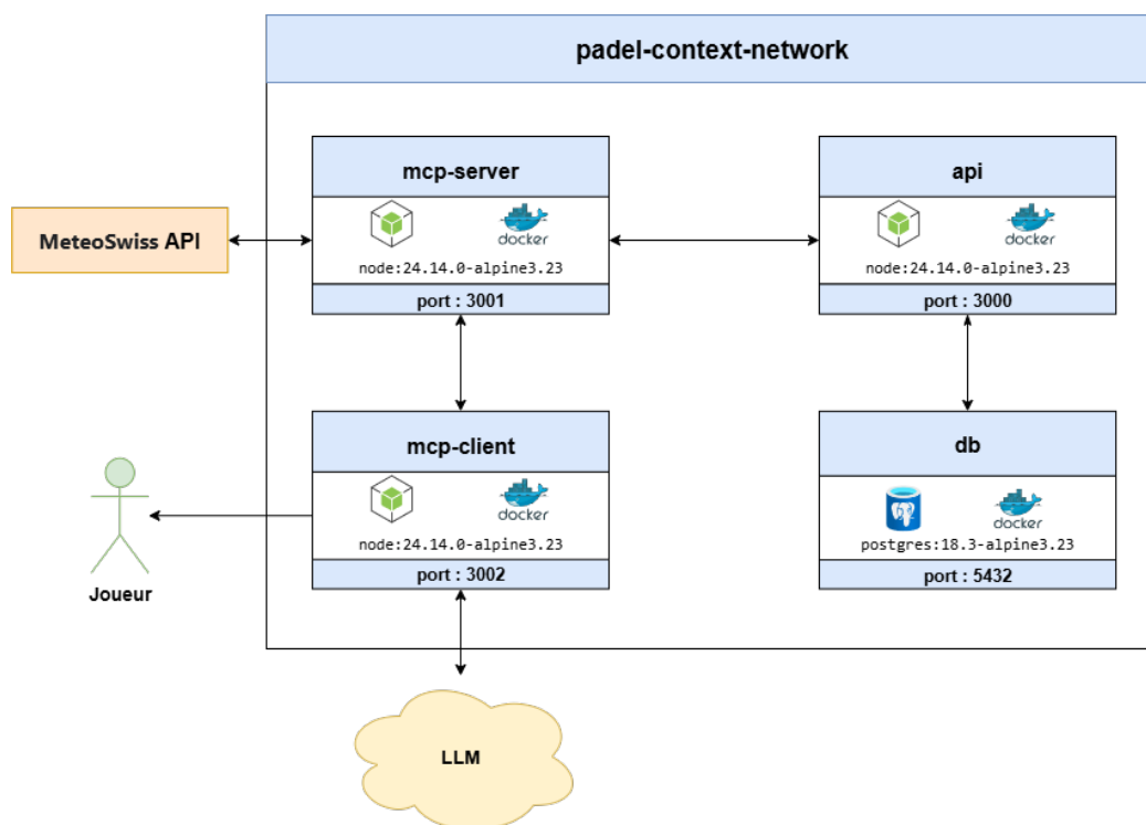
FIGURE 5 – Diagramme de l'architecture logicielle de l'écosystème Padel-Context
