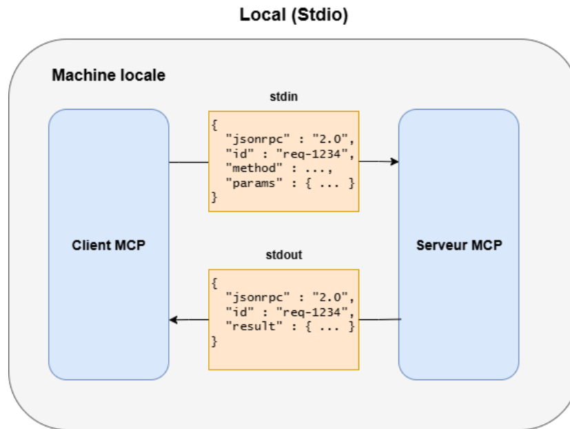
FIGURE 6 – Mécanisme de transport local via Stdio, adapté de (Dohnal, 2025) [15]
