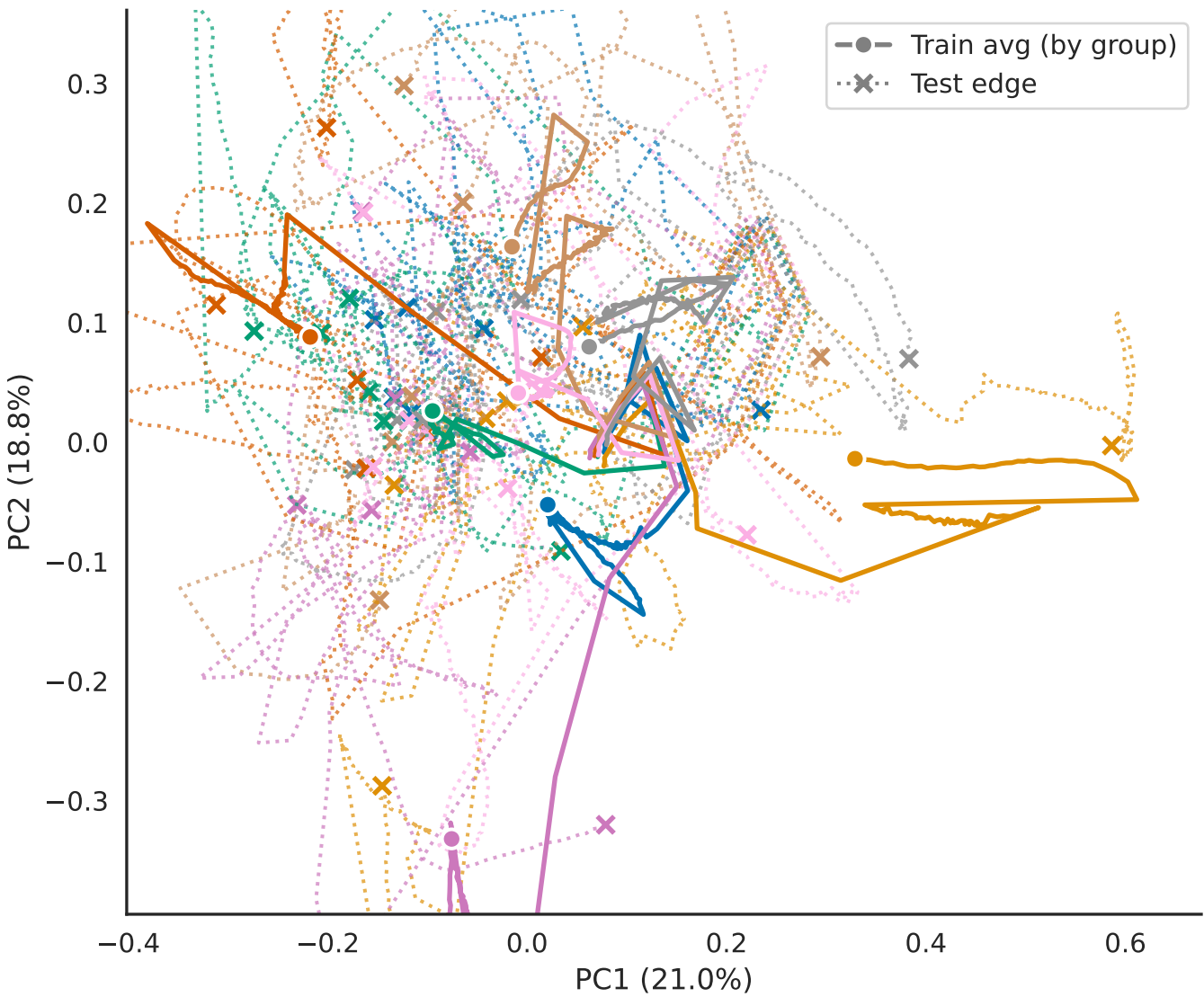
Residual PCA trails
