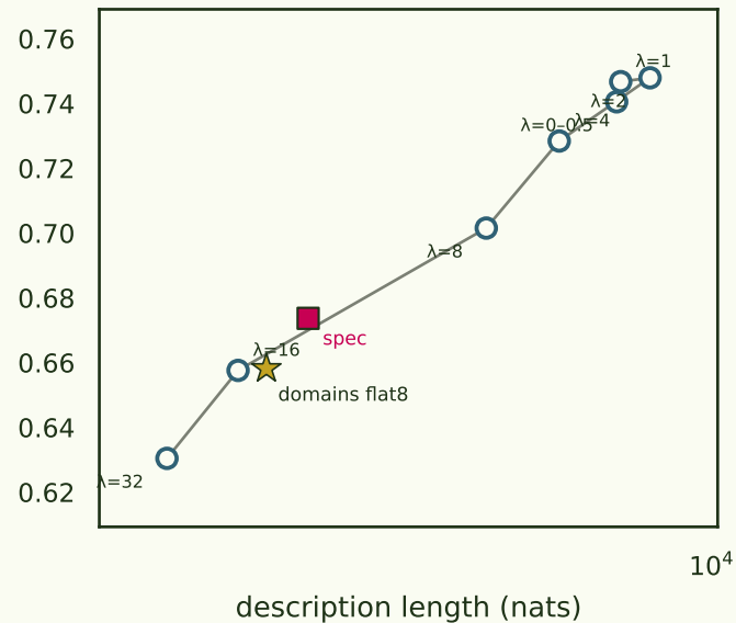
Pythia/Pile seed 0 (n=400)
