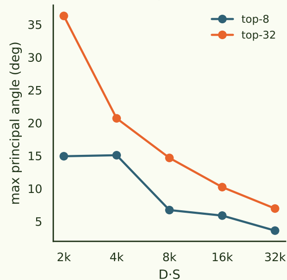
eigenspace error
