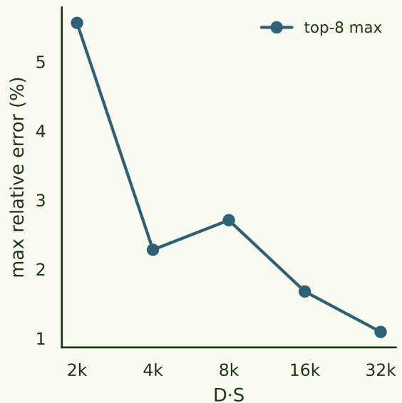
eigenvalues
