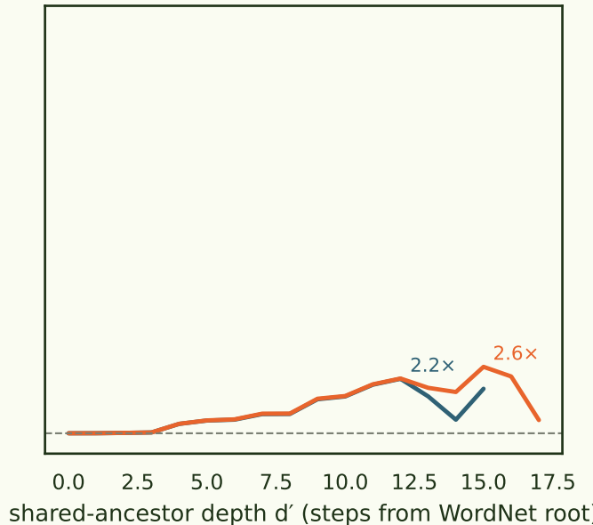
ImageGPT-small (label-free loss)
