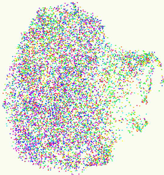
ImageGPT-small
