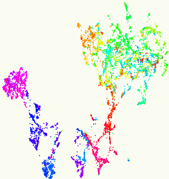
Inception-v1
