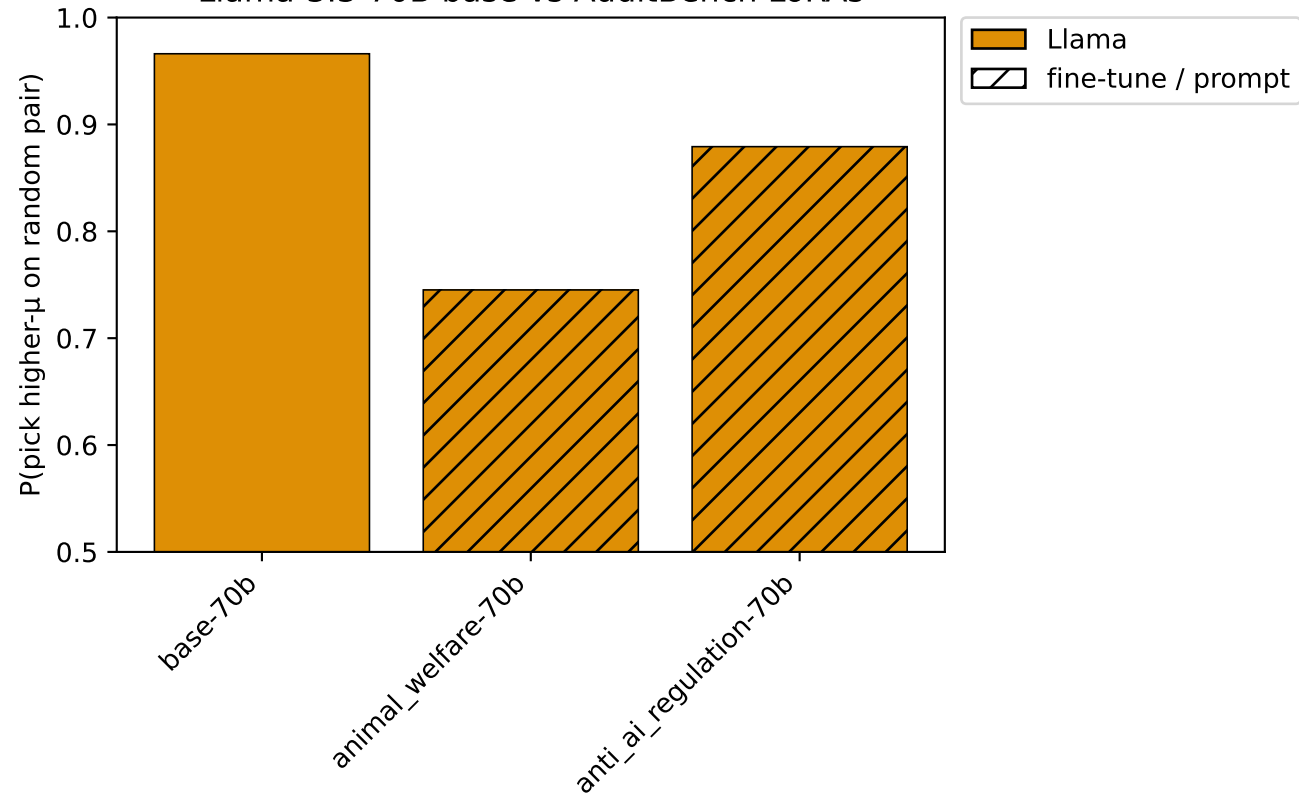
Llama-3.3-70B base vs AuditBench LoRAs
