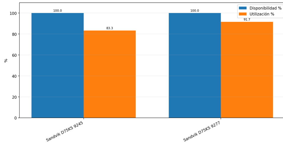
Disponibilidad y utilización promedio por equipo
