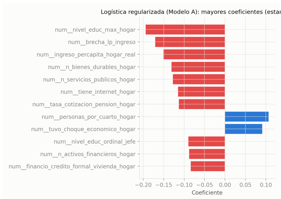
Figura 14: Mayores coeficientes en valor absoluto, regresión logística regularizada, Modelo A (unidades estandarizadas).
