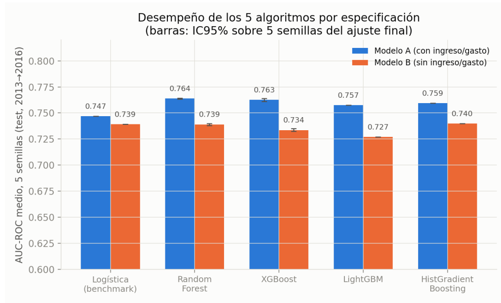
Figura 11: AUC-ROC medio (5 semillas) de los cinco algoritmos por especificación, conjunto de prueba 2013→2016. Barras de error: IC95 %.
