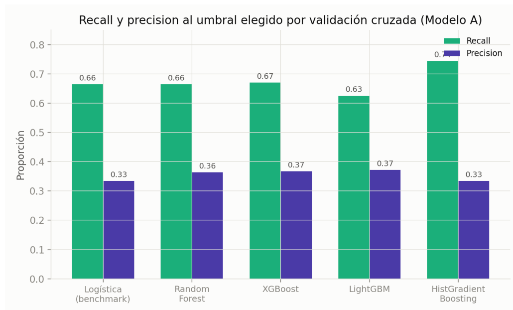
Figura 8: Recall y precision al umbral de clasificación elegido por validación cruzada, Modelo A.
