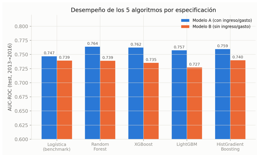
Figura 7: AUC-ROC de los cinco algoritmos por especificación, conjunto de prueba 2013→2016.
