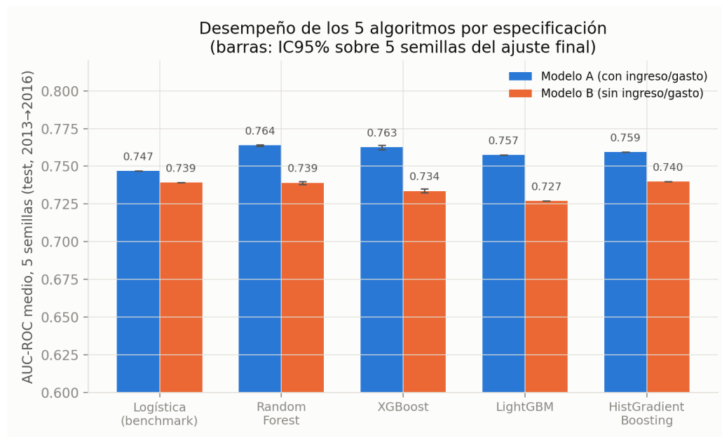
Figura 19: AUC-ROC medio (5 semillas) de los cinco algoritmos por especificación, conjunto de prueba 2013→2016. Barras de error: IC95 %.
