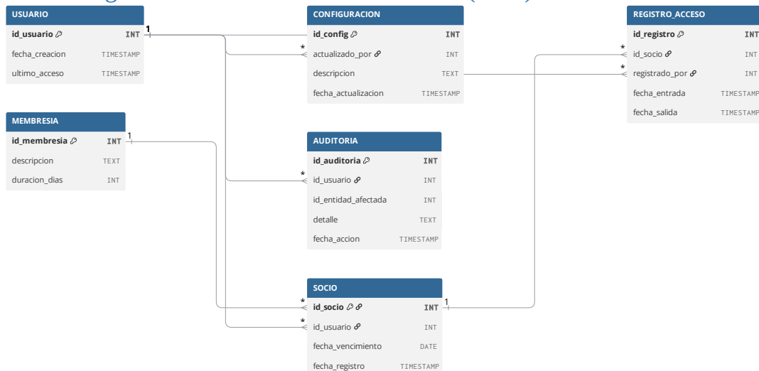
Ilustración 9 Diagrama ENTIDAD-RELACION
