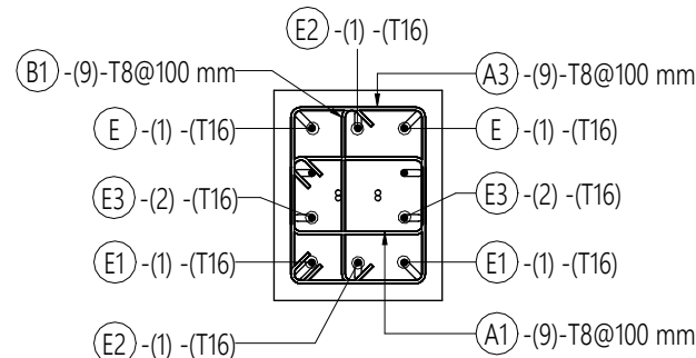
2 SECTION (REINF) 1 : 20
