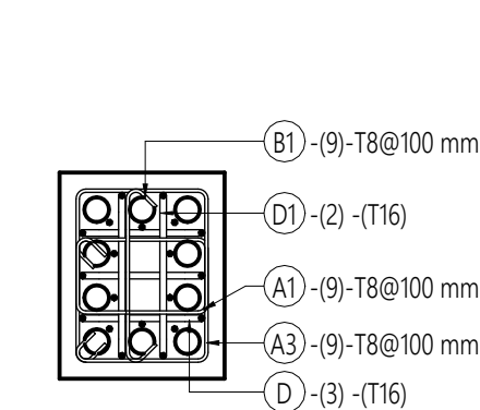
1 SECTION (REINF) 1 : 20
