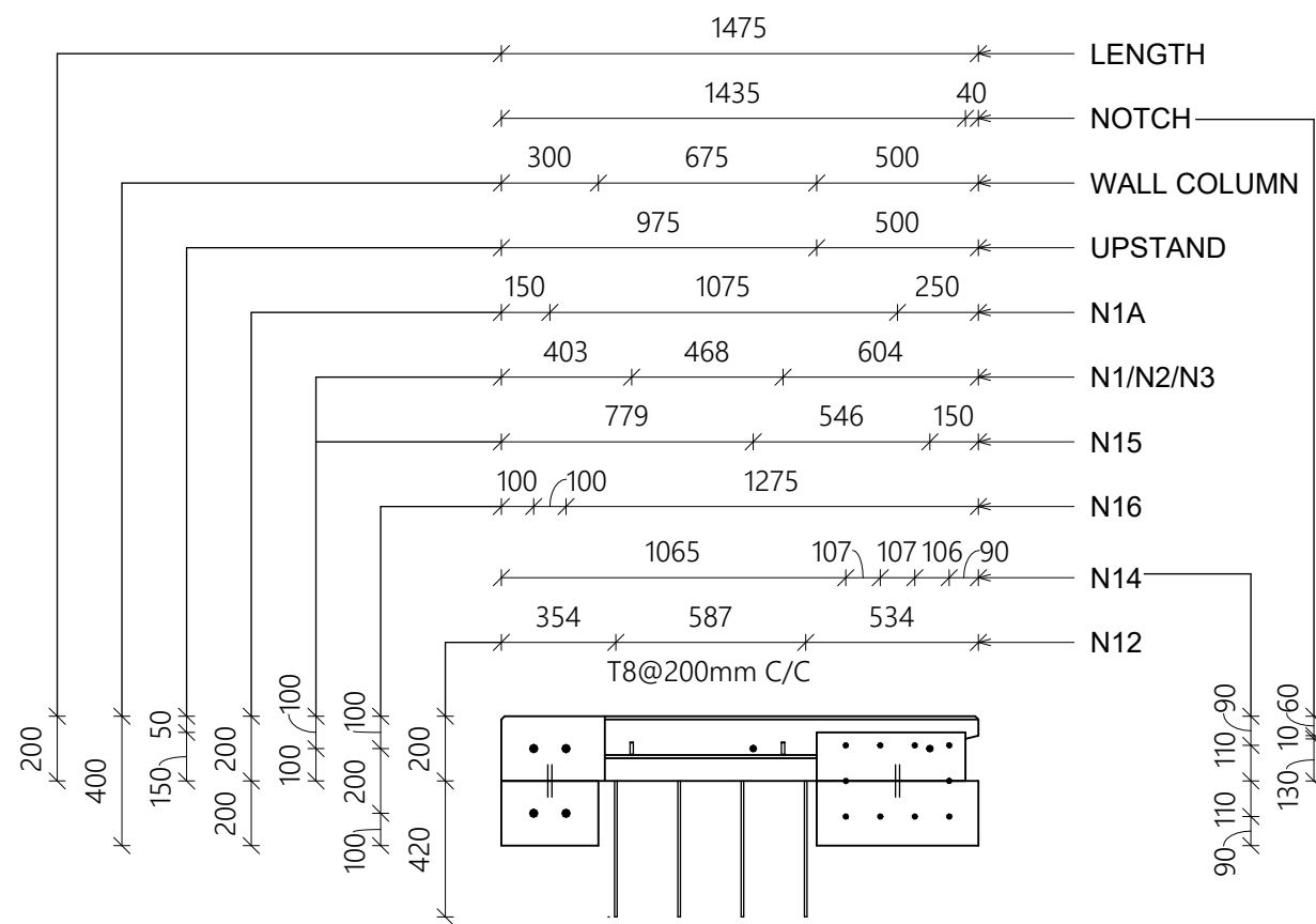
4 SECTION 1 : 25
