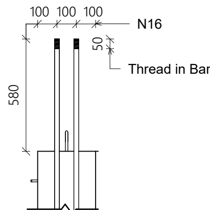
6 DETAIL 1 : 20
