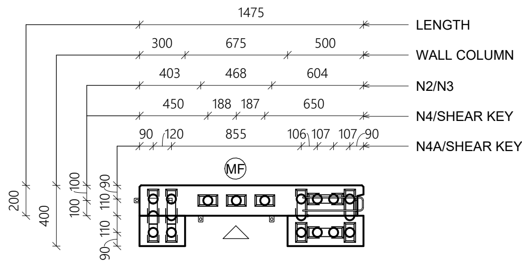
5 SECTION 1 : 25
