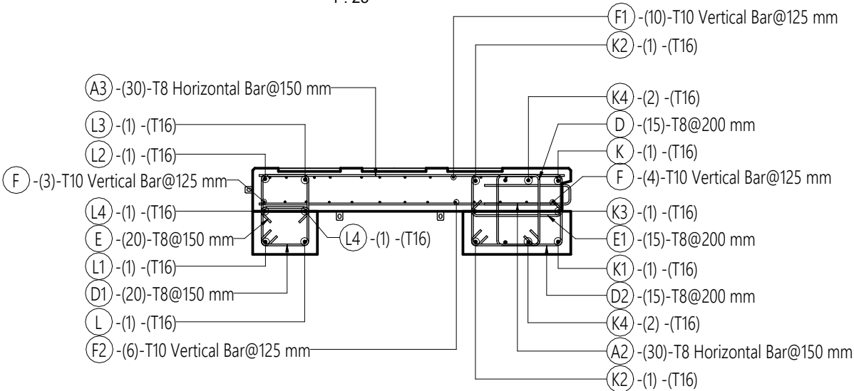
5 SECTION (REINF) 1 : 25
