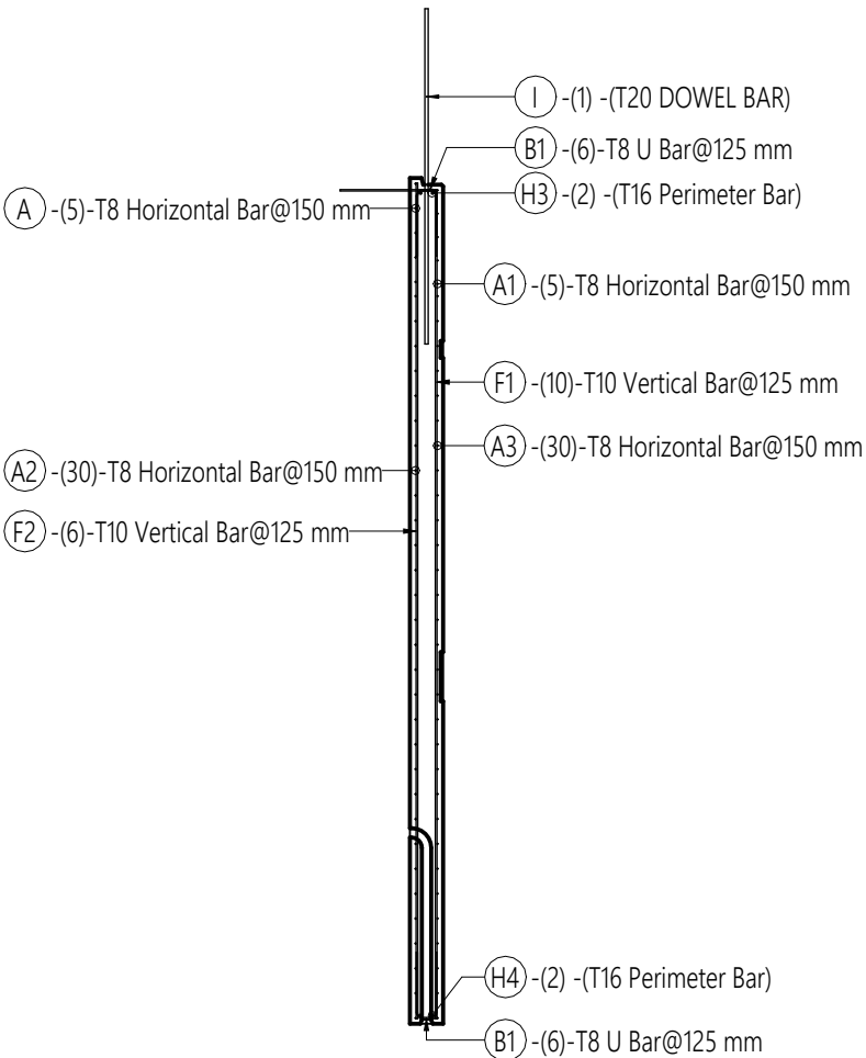
2 SECTION (REINF) 1 : 50
