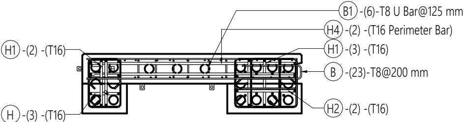
6 SECTION (REINF) 1 : 25
