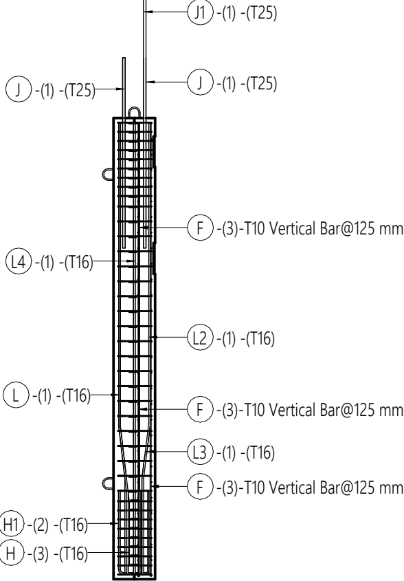
3 SECTION (REINF) 1 : 50
