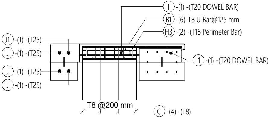
4 SECTION (REINF) 1 : 25
