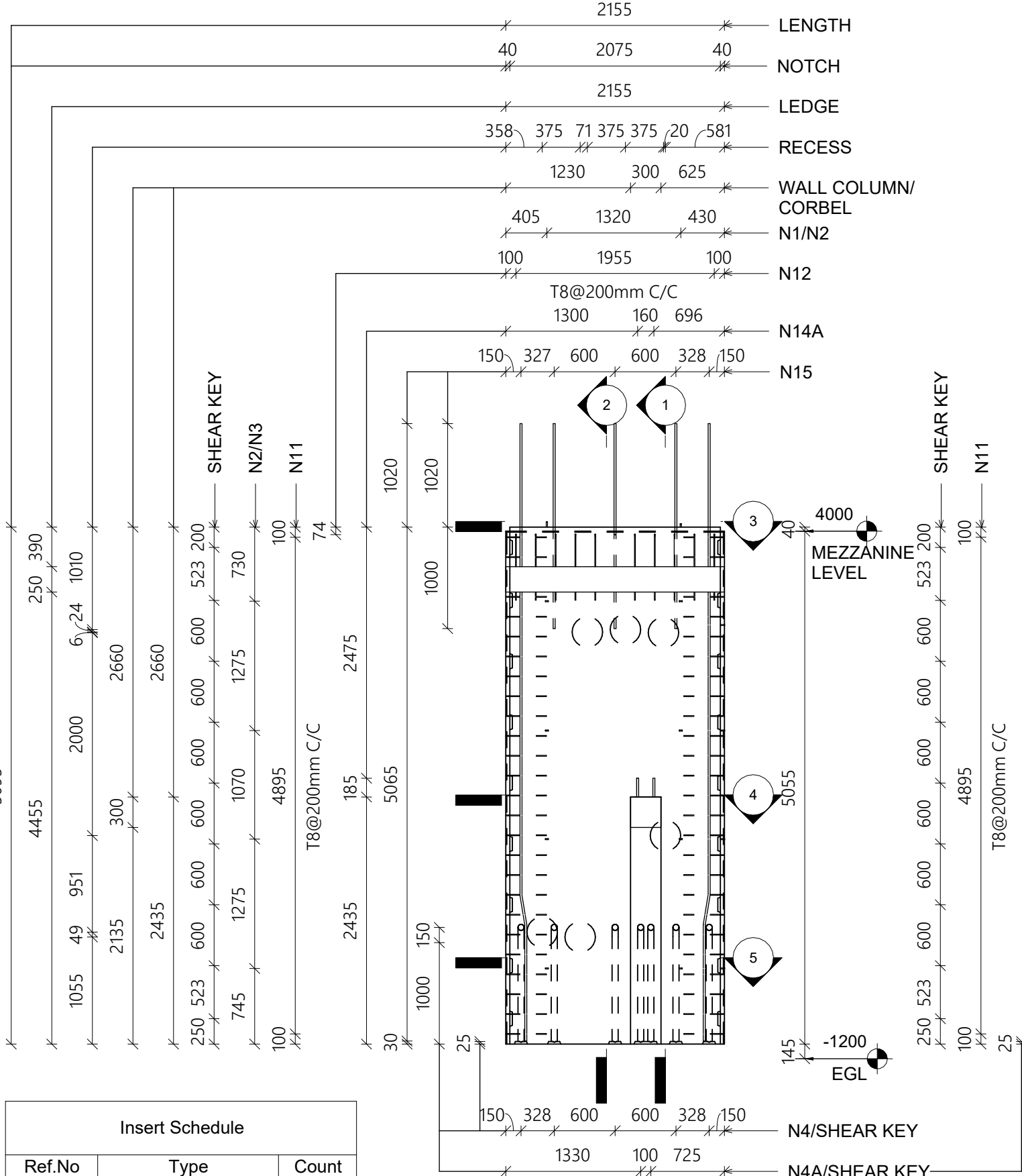
A ELEVATION 1 : 50
