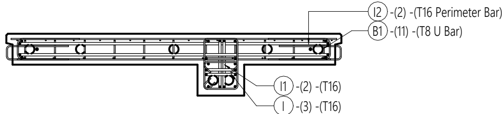
5 SECTION (REINF) 1 : 25
