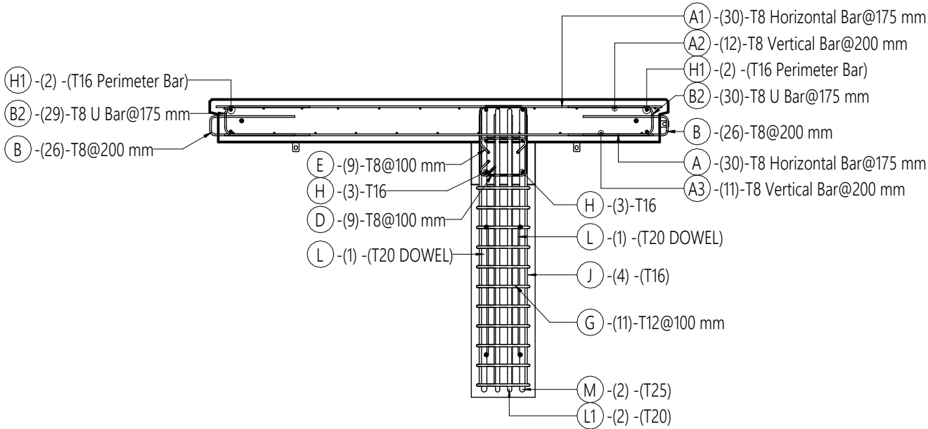
4 SECTION (REINF) 1 : 25
