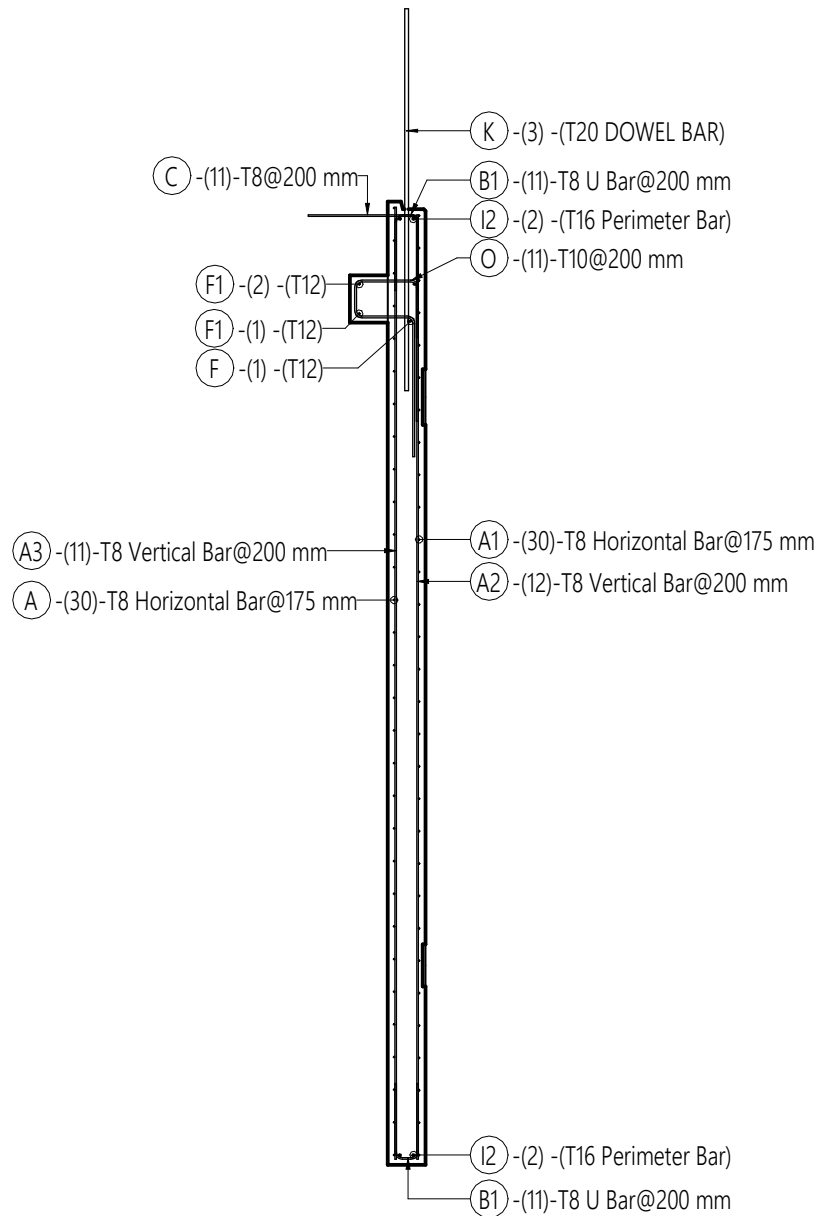
2 SECTION (REINF) 1 : 40
