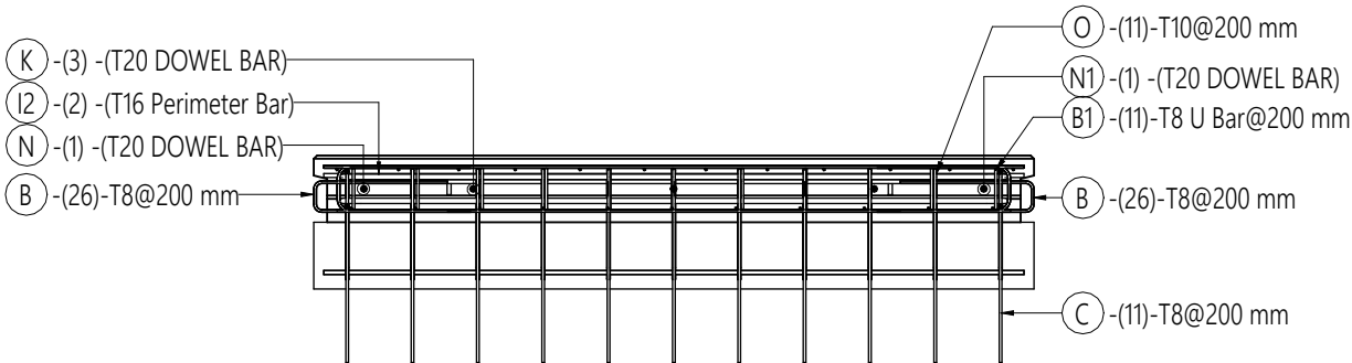
3 SECTION (REINF) 1 : 25
