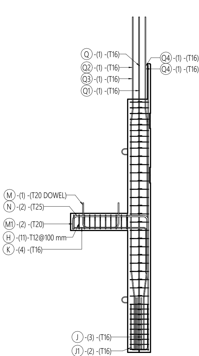
2 SECTION (REINF) 1 : 40
