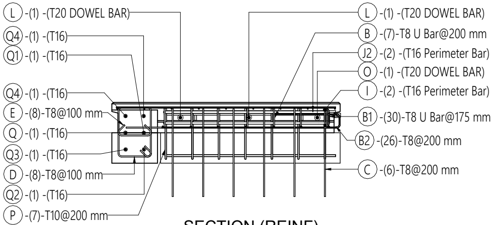
3 SECTION (REINF) 1 : 25
