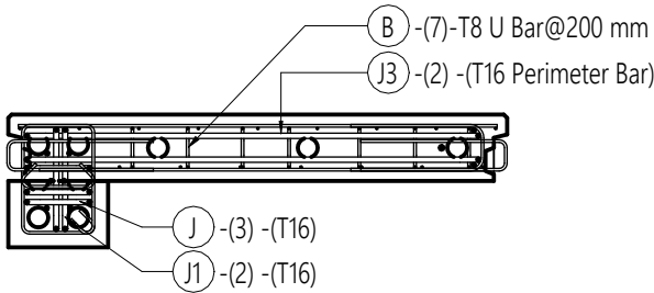
5 SECTION (REINF) 1 : 25
