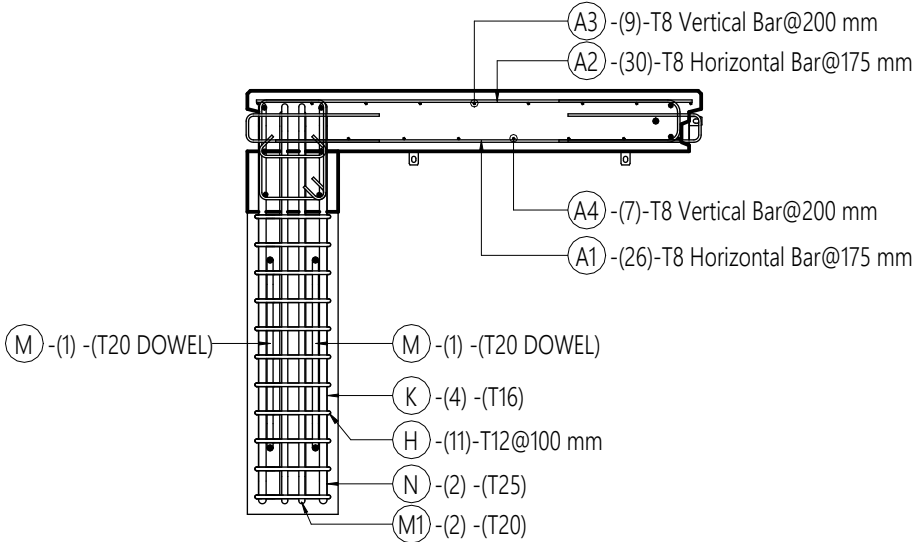
4 SECTION (REINF) 1 : 25
