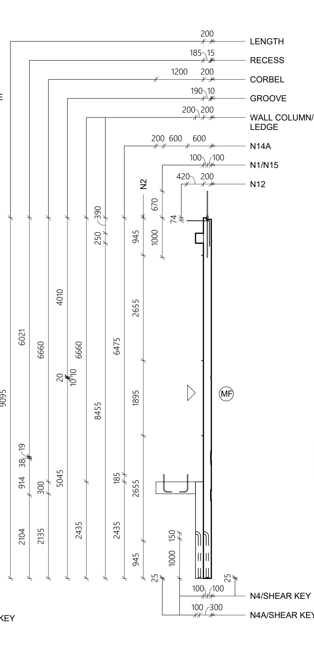
B SECTION 1 : 60
