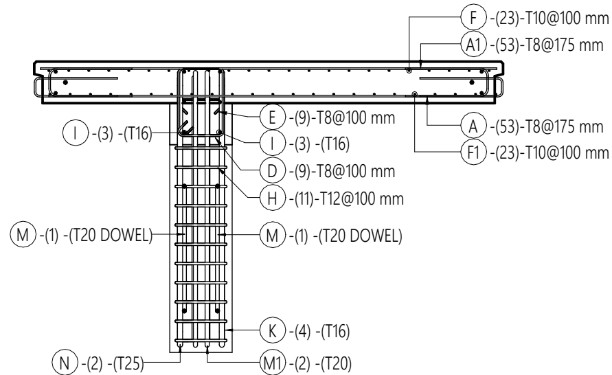
4 SECTION (REINF) 1 : 25
