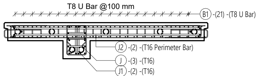
5 SECTION (REINF) 1 : 25
