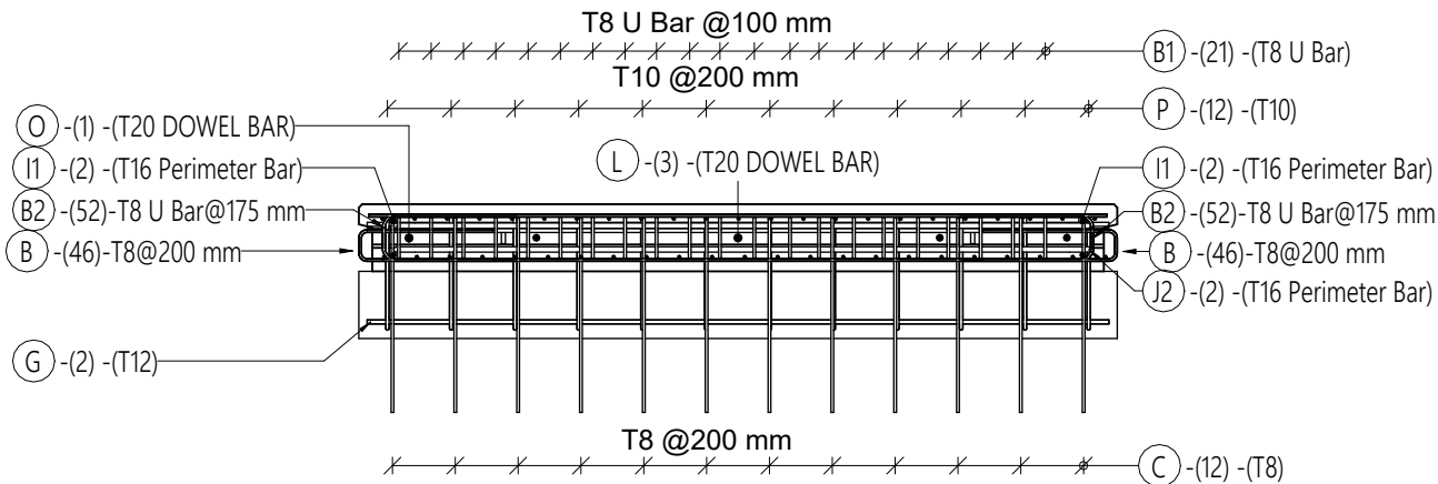
3 SECTION (REINF) 1 : 25
